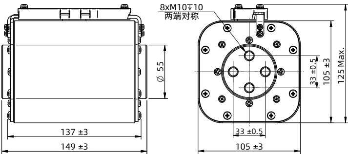
尺寸 (mm)
